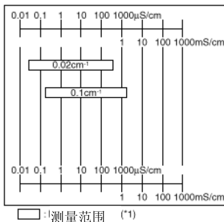
图 2 电极常数与测量范围的关系
