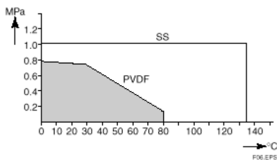
图 1 温度和压力的容许范围
